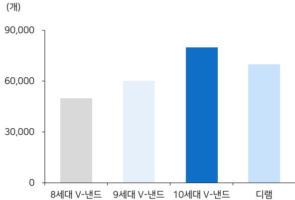
그림3 프로브카드 핀 수 비교
