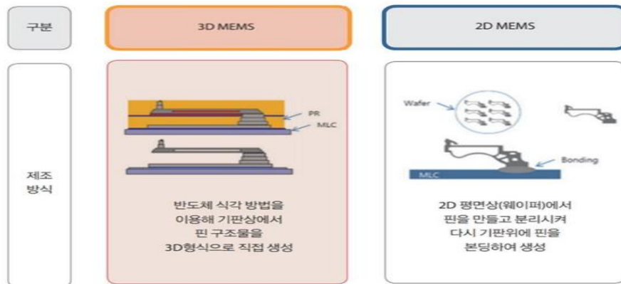
그림1 3D MemS vs 2D MemS 프로브카드 제작 방식 비교
