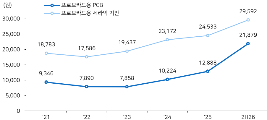
그림5 프로브카드 주요 원재료 가격 추이
