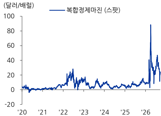
도표4. 복합정제마진
