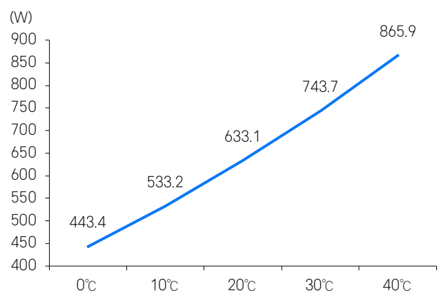
라디에이터의 온도별 복사열 배출량
