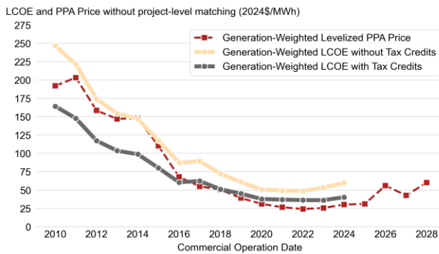
그림 8. 태양광 LCOE/PPA 가격 추이 (1)
