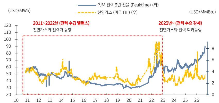
그림 14. 미국 전력 구매가격 vs. 천연가스 (동행 → 디커플링)
