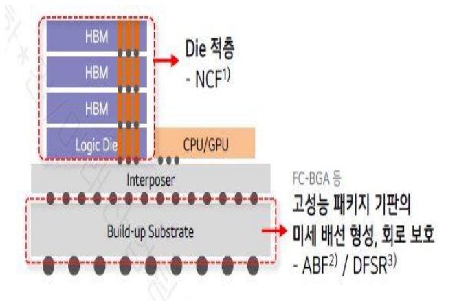
도표 9. 진공 라미네이터 솔루션
