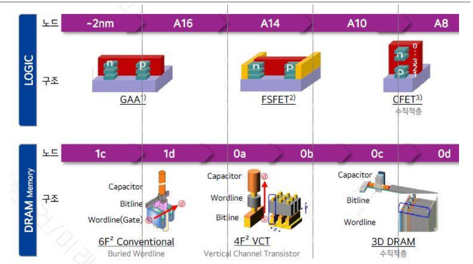
도표 5. 3D DRAM 구조 전환_고정밀/고다층 Epitaxy
