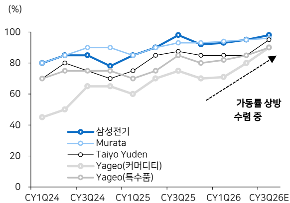
그림23 주요 MLCC 업체들 가동률 비교
