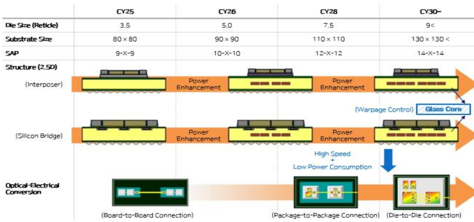
그림27 ABF 기판 기술 로드맵
