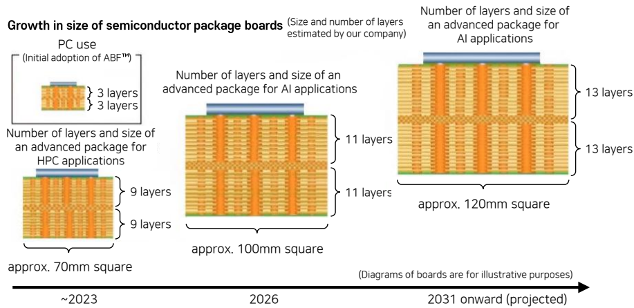
그림26 ABF 기판 스펙 발전 추이 및 전망
