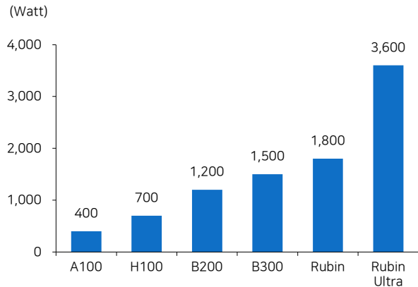
그림20 칩 1개당 전력 소모량 비교
