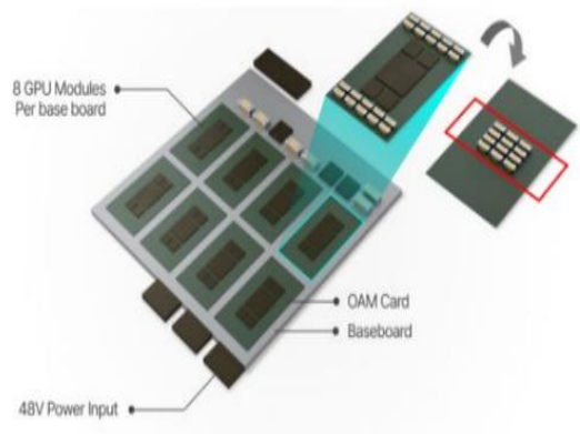
그림10 커패시터는 GPU와 인접한 배치 요구 → 소형화 필수
