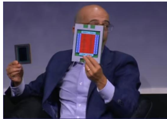
그림31 반도체 칩 고성능화에 따른 ABF 기판의 대면적화 (4)
