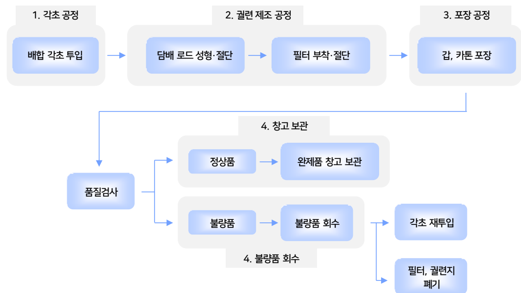
그림8 결련 담배 제조 공정
