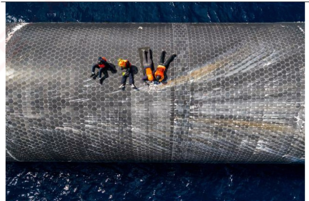
[그림 5] 해상에서 진행된 Ship 40의 열차폐 타일 점검
