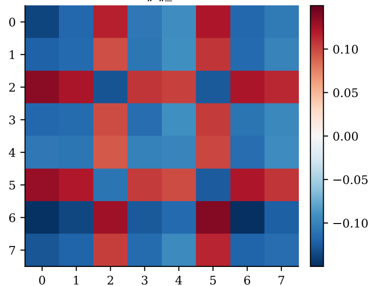
U^T V ( \|\cdot\|_F=0.918 )
