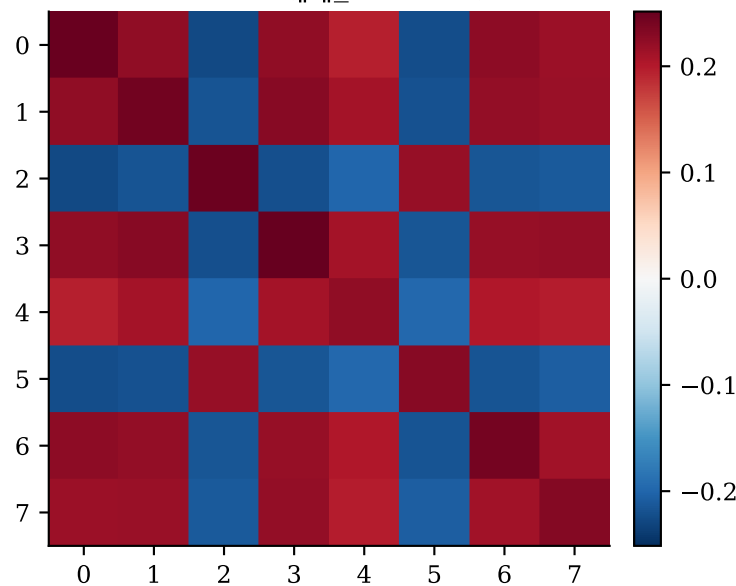
V^T V ( \|\cdot\|_F=1.744 )
