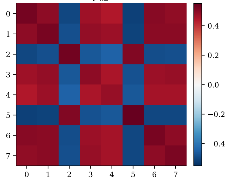
U^T U ( \|\cdot\|_F=3.896 )
