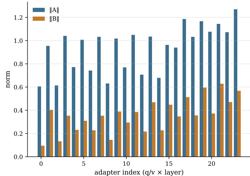
r=1 (Phase 1) per-adapter A/B norm ( \|A\|_{\text{tot}}=4.68 , \|B\|_{\text{tot}}=1.87 )
