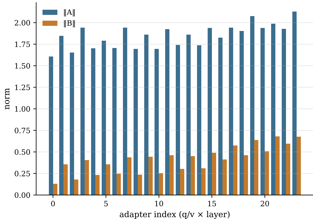
r=8 (Phase 2b) per-adapter A/B norm ( \|A\|_{\text{tot}}=9.07 , \|B\|_{\text{tot}}=2.13 )
