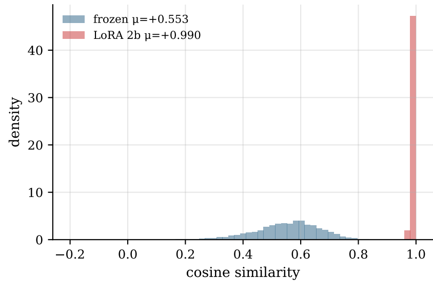
nfcopus — random token-pair cosine
