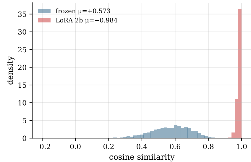
scifact — random token-pair cosine
