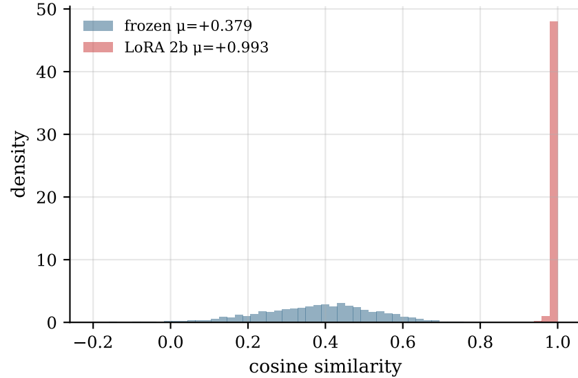
fiqa — random token-pair cosine
