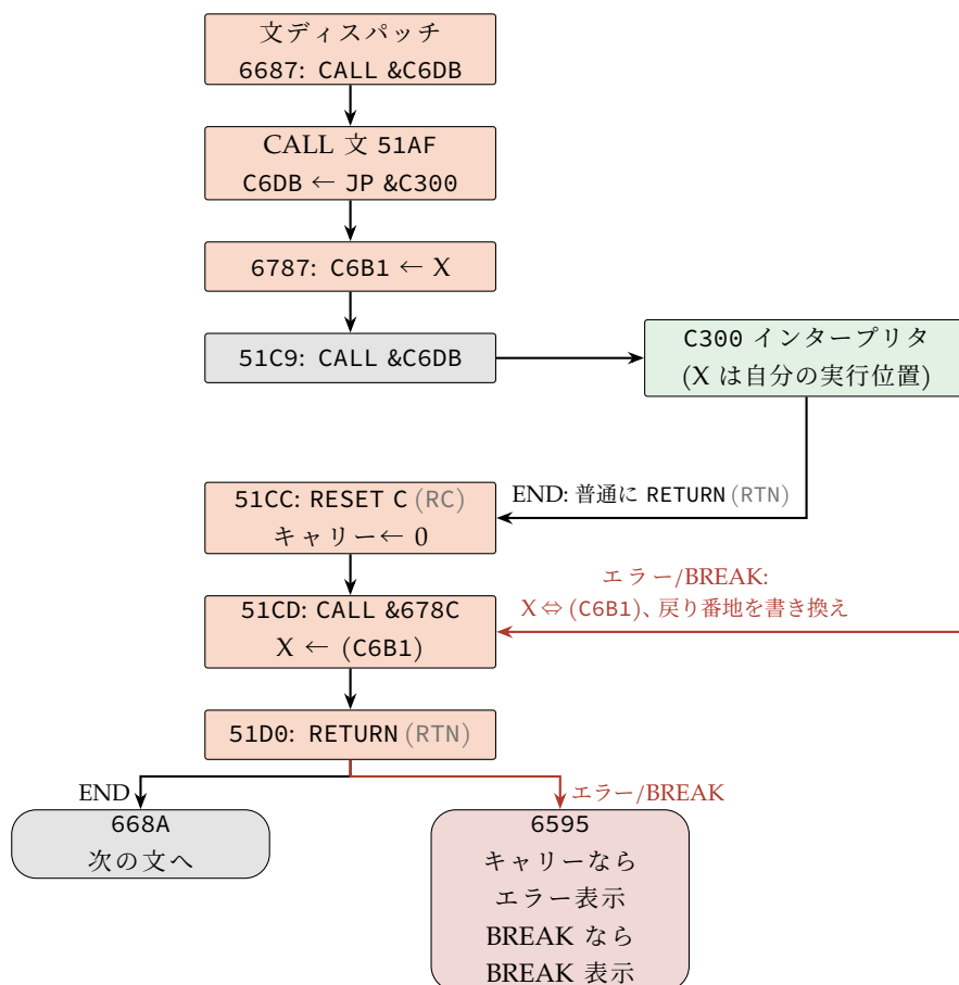
図 1.9 BASIC の CALL 文からインタープリタに入り、BASIC に戻るまで (番地は PC-1251 の ROM)
