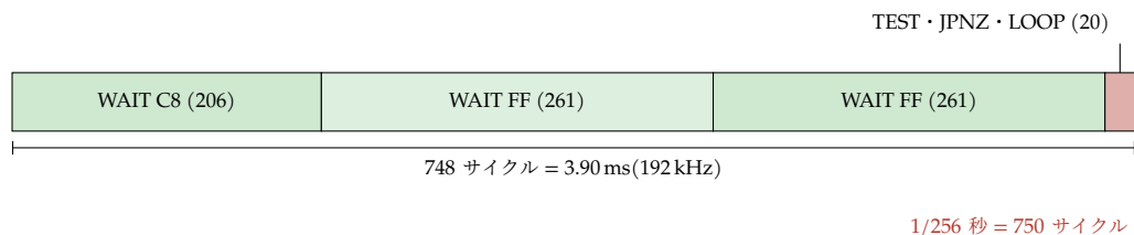
図 3.10 WAIT の内側ループ 1 周の内訳 (utz82 のサイクル表による)
