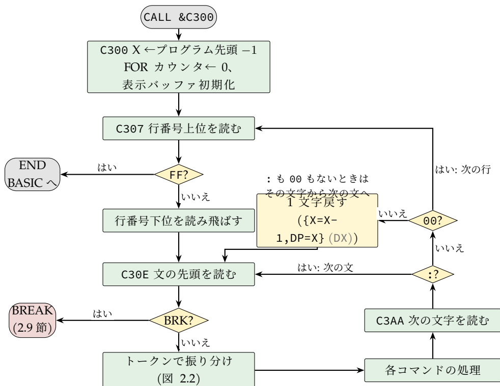
図 2.1 メインループ
