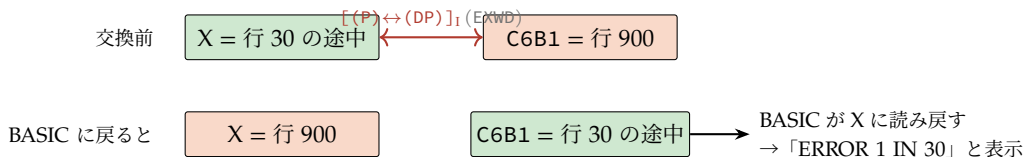
図 3.11 実行位置の交換。BASIC は行 30 で自分がエラーを起こしたと受け取る
