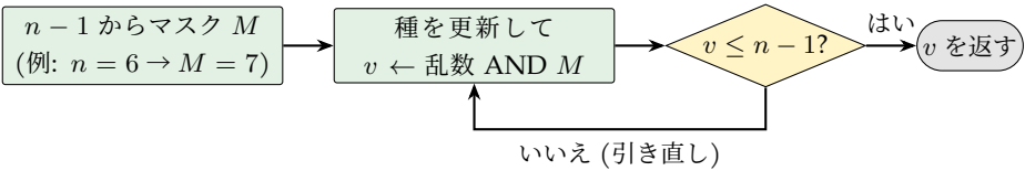
図 2.13 RND の手順
