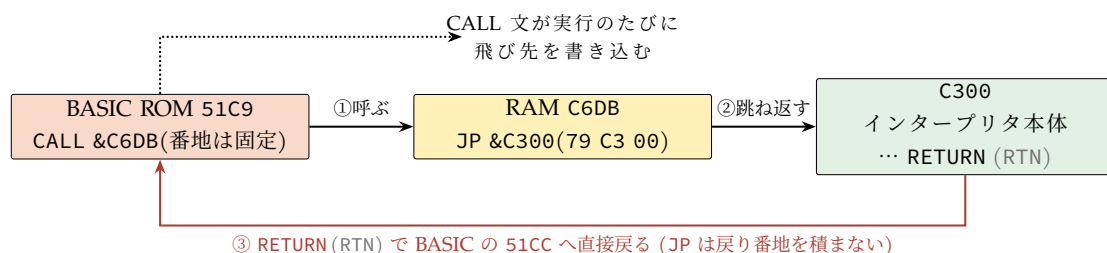
図 1.3 トランポリン。BASIC は固定の番地 C6DB を呼び、そこに書いた JP が本当の飛び先へ跳ね返す
