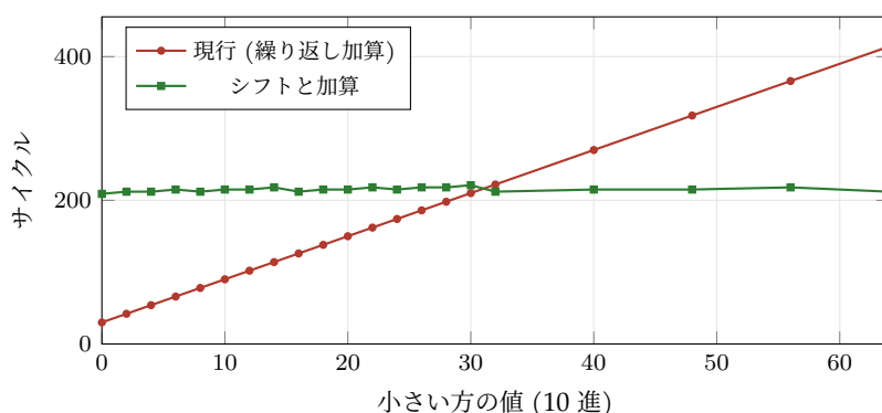
図 4.2 掛け算の所要サイクル (実測)。FF*FF では現行 1560、シフト 233
