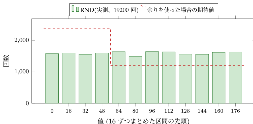
図 3.9 RND C0 の分布。棄却法では各区間がほぼ 1600 回で揃う
