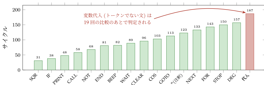
図 4.1 文の先頭を読んでから処理ルーチンに着くまでのサイクル数 (実測)。右端の赤が変数代入
