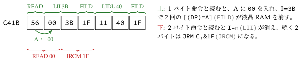
図 1.5 COS(画面消去) の先頭。56 の長さで命令の区切りが変わる
