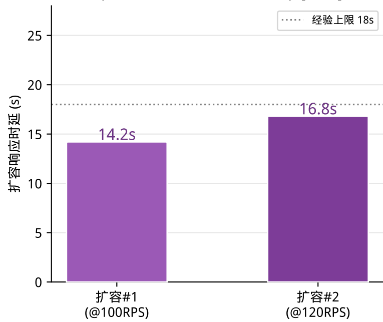
(C) 横向扩容响应时延 (进程启动至首次推理就绪) [实测]
