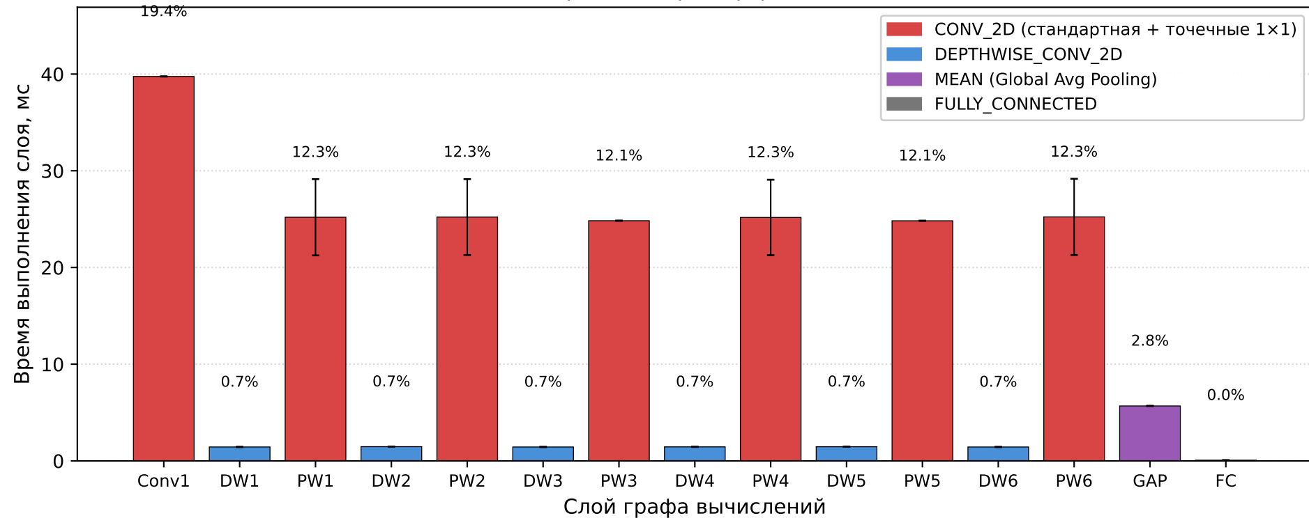
Распределение времени инференса DS-CNN по слоям на ESP32-S3 (n=100 прогонов, ср. инференс = 205 мс)
