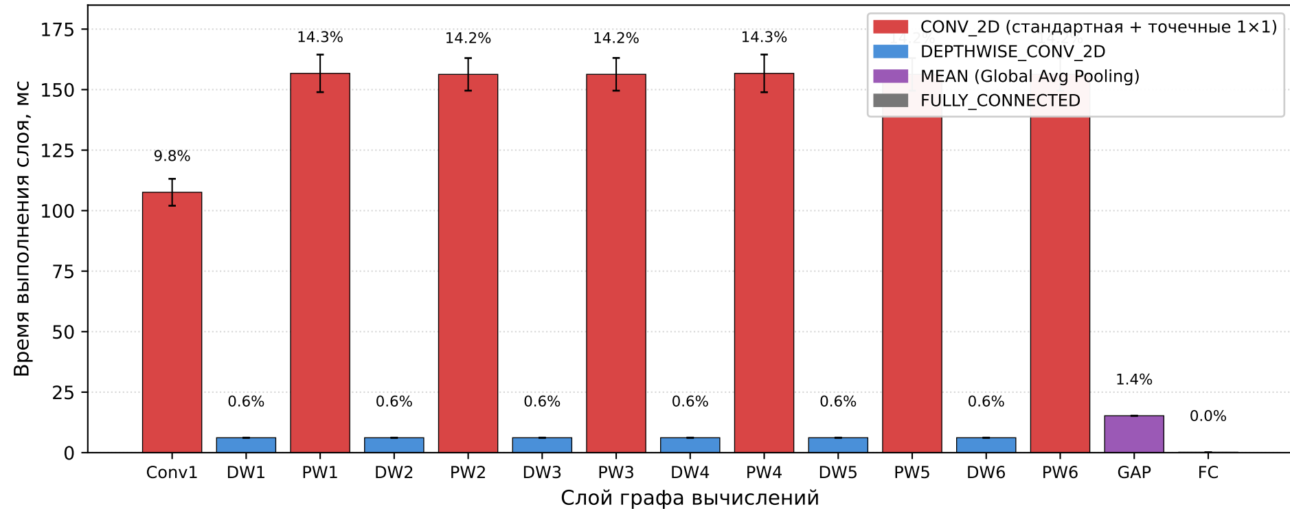
Распределение времени инференса DS-CNN по слоям на ESP32-S3 (n=100 прогонов, ср. инференс = 1099 мс)
