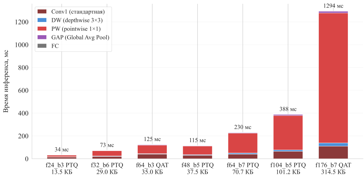
Рисунок 10 — Послойная декомпозиция времени инференса DS-CNN на ESP32-S3 для архитектур различного размера, абсолютные значения
