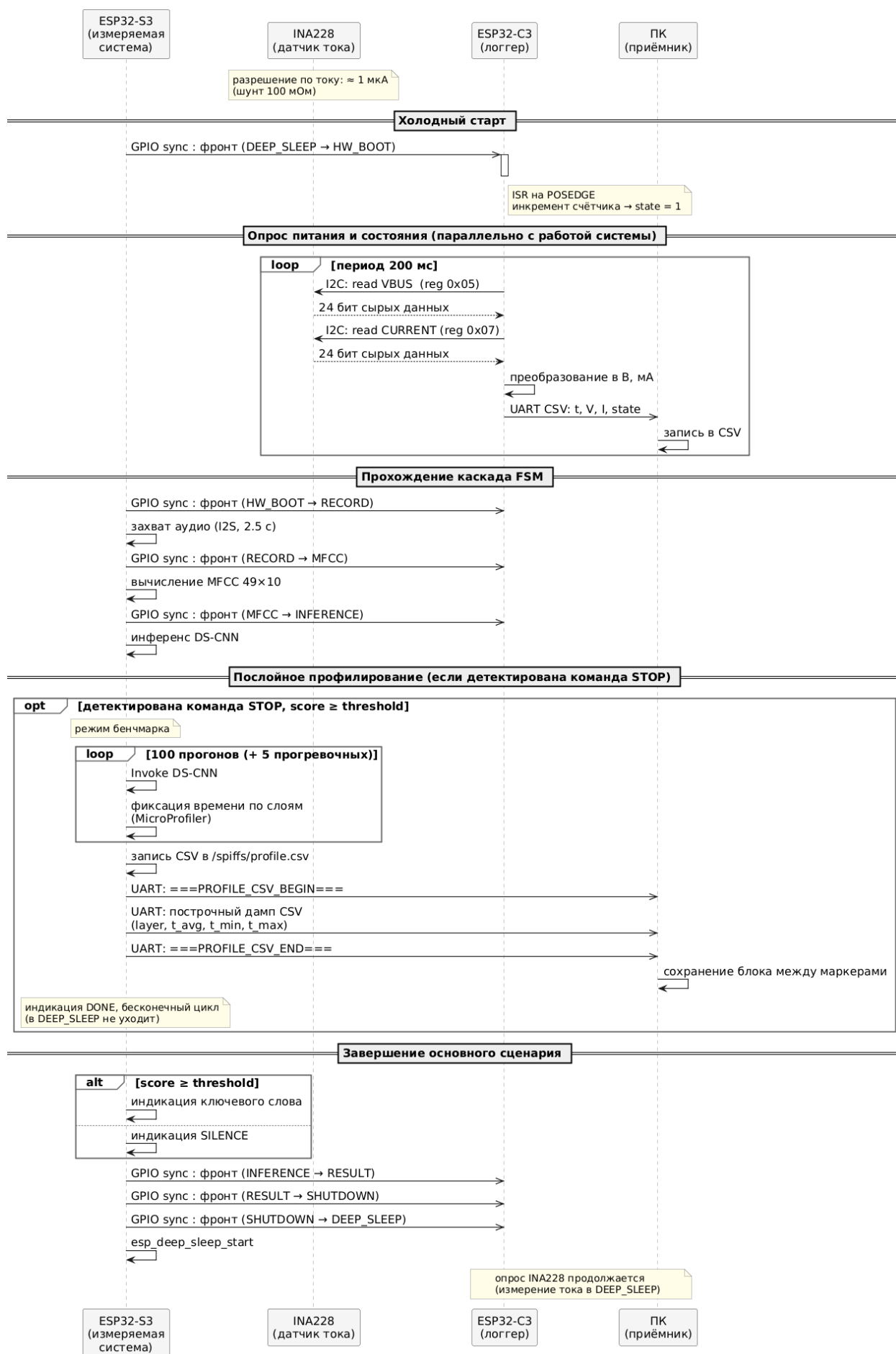
Рисунок 23 — Диаграмма последовательности сбора измерительных данных 108
