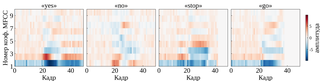
Рисунок 5 — Матрицы MFCC-признаков для четырёх ключевых слов из набора Google Speech Commands: «yes», «no», «stop», «go»
