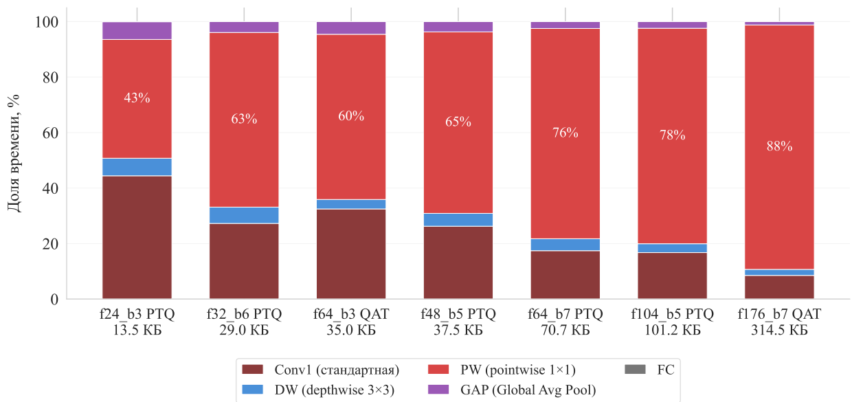
Рисунок 11 — Послойная декомпозиция времени инференса DS-CNN на ESP32-S3 для архитектур различного размера, относительные доли
