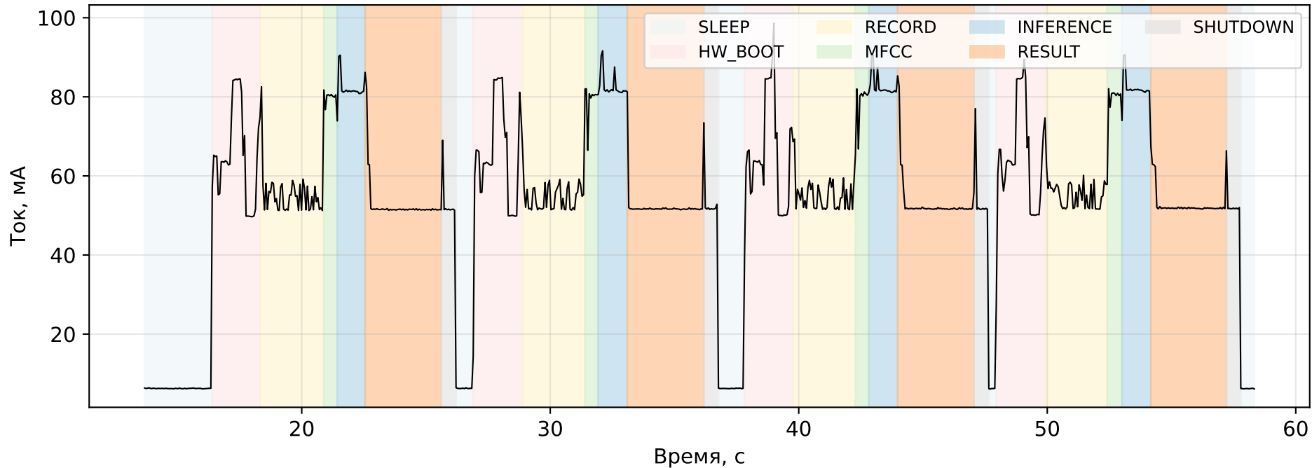
Профиль тока полного цикла каскадной обработки
