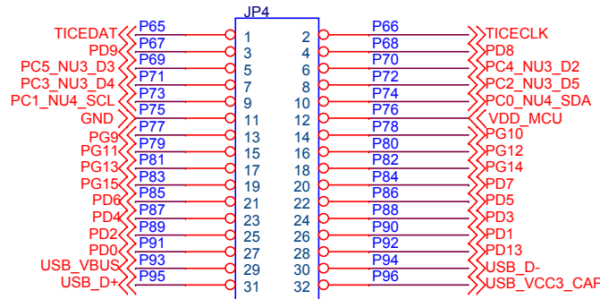
HEADER 2.54 16X2 male(NC)
