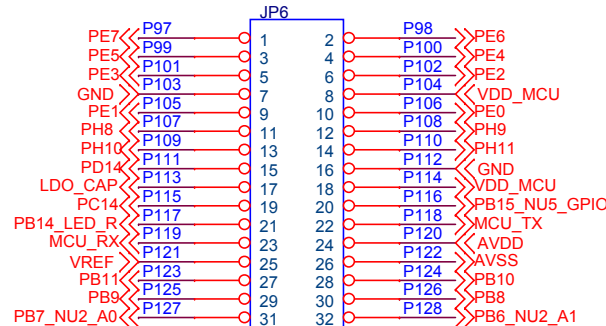
HEADER 2.54 16X2 male(NC)
