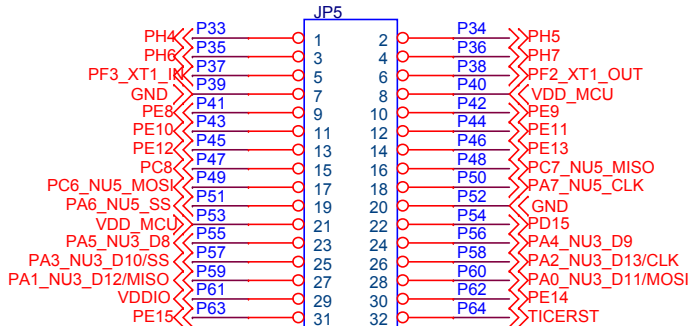
HEADER 2.54 16X2 male(NC)
