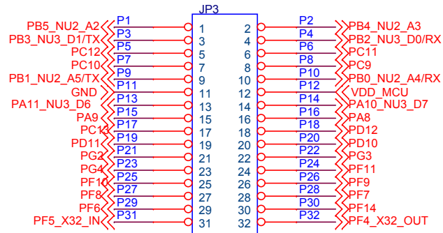
HEADER 2.54 16X2 male(NC)
