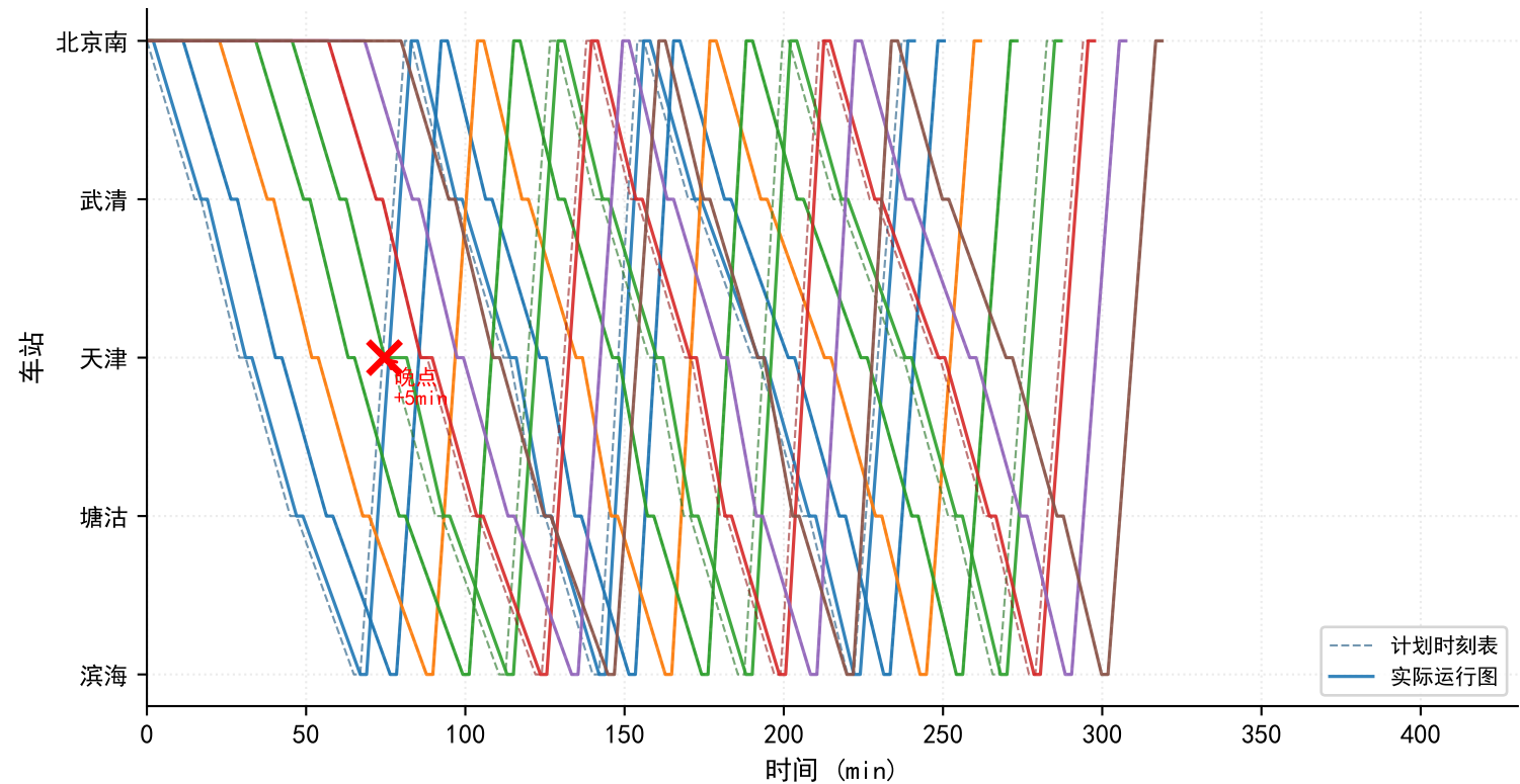
(c) 常规场景 — 鲁棒模型预测控制
