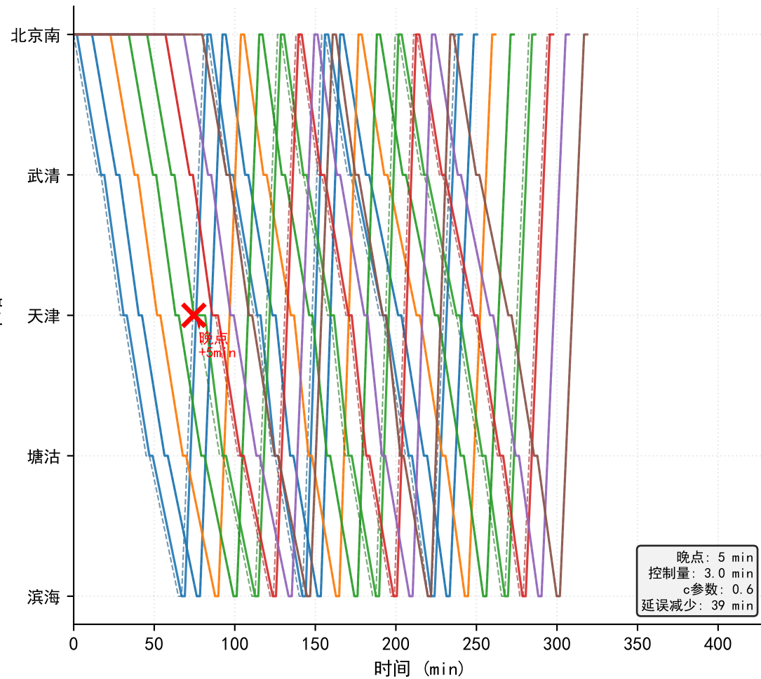
(a) 紧急场景 — 反馈控制
