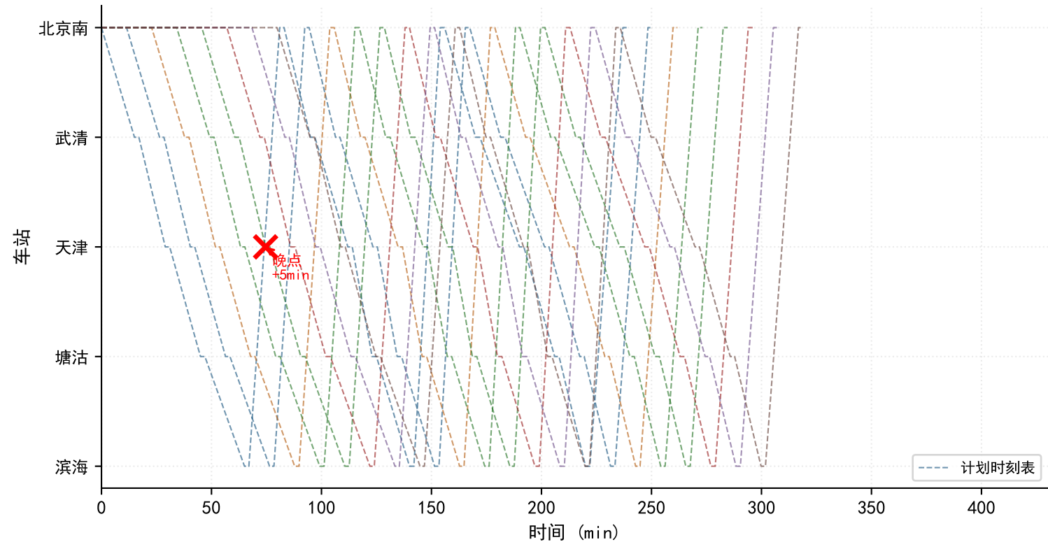
无控制策略（FCFS）—— RMPC场景
