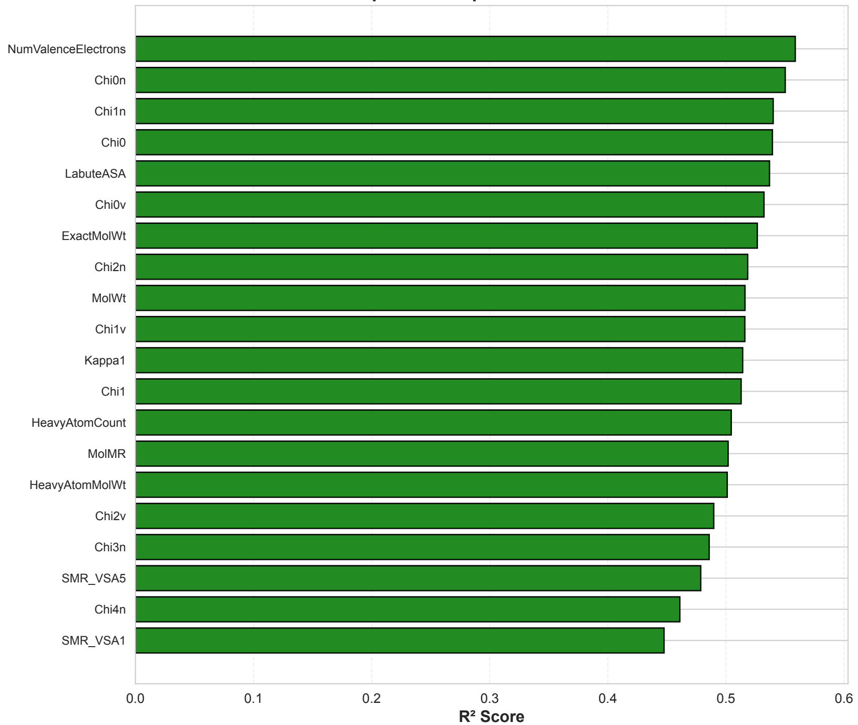
Top 20 Descriptors - MLP Probe
