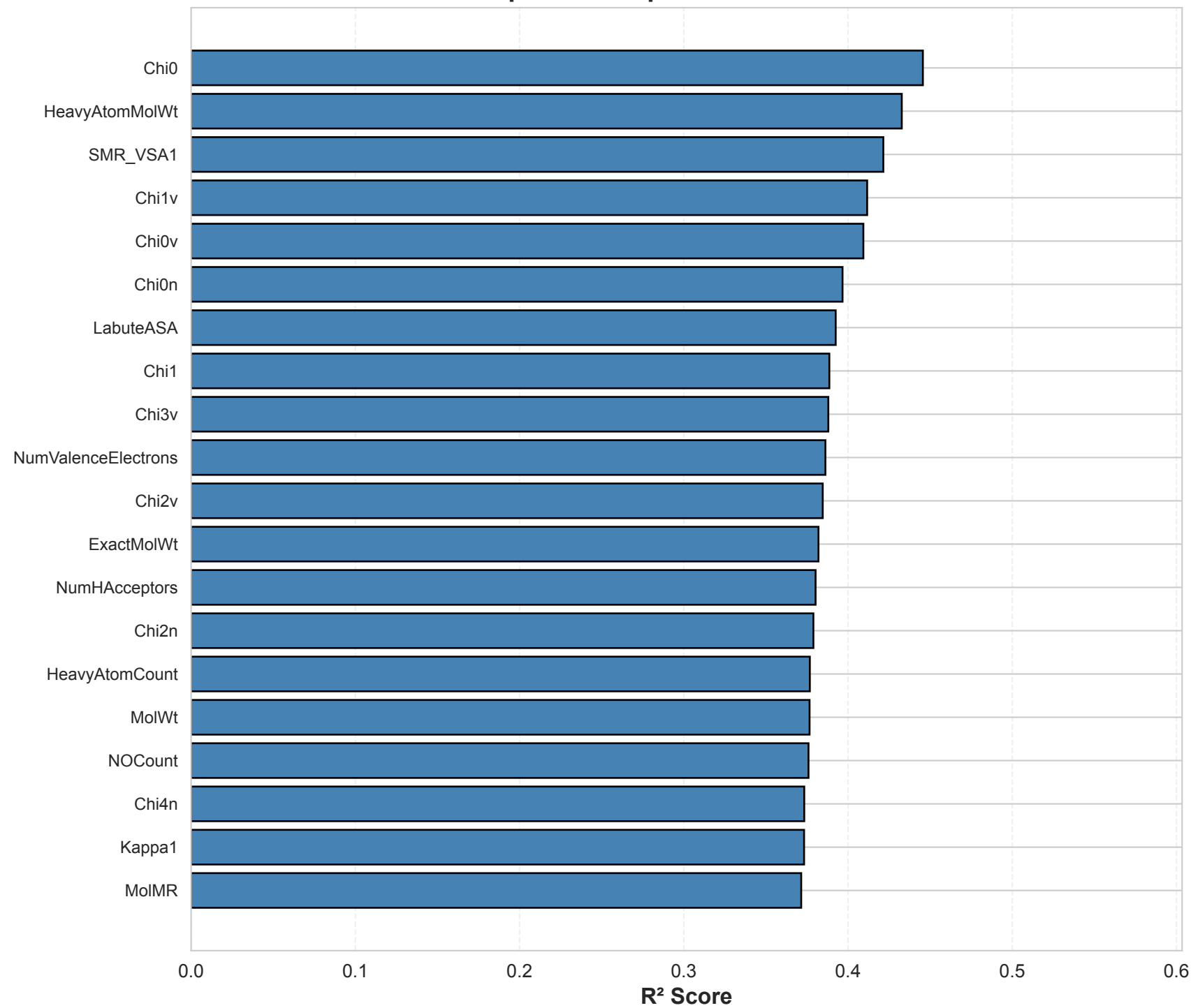
Top 20 Descriptors - Linear Probe
