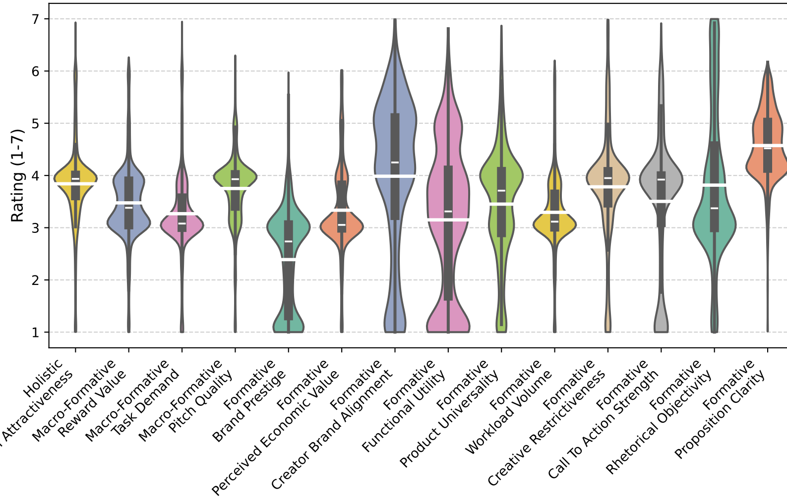
Model: Gemma 4
