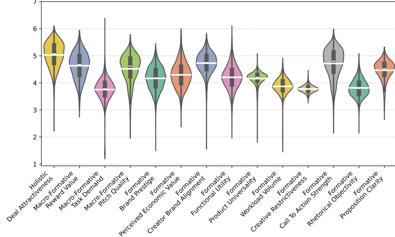
Model: Llama 3.2
