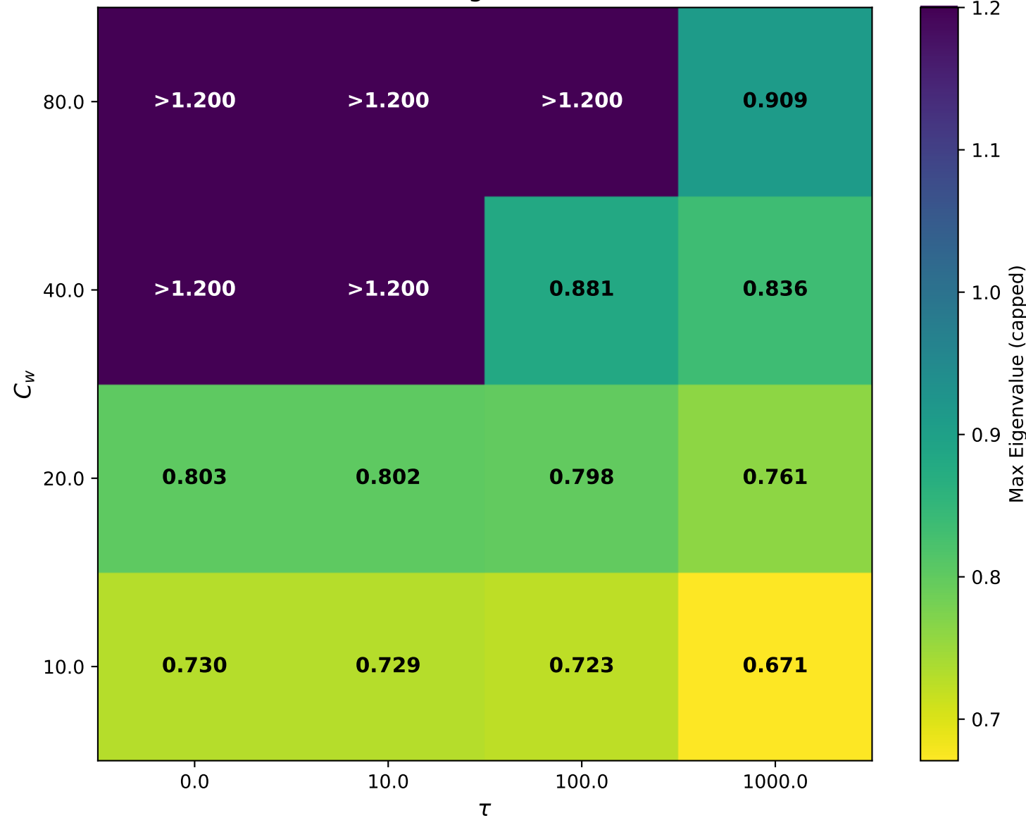
Max Eigenvalue
