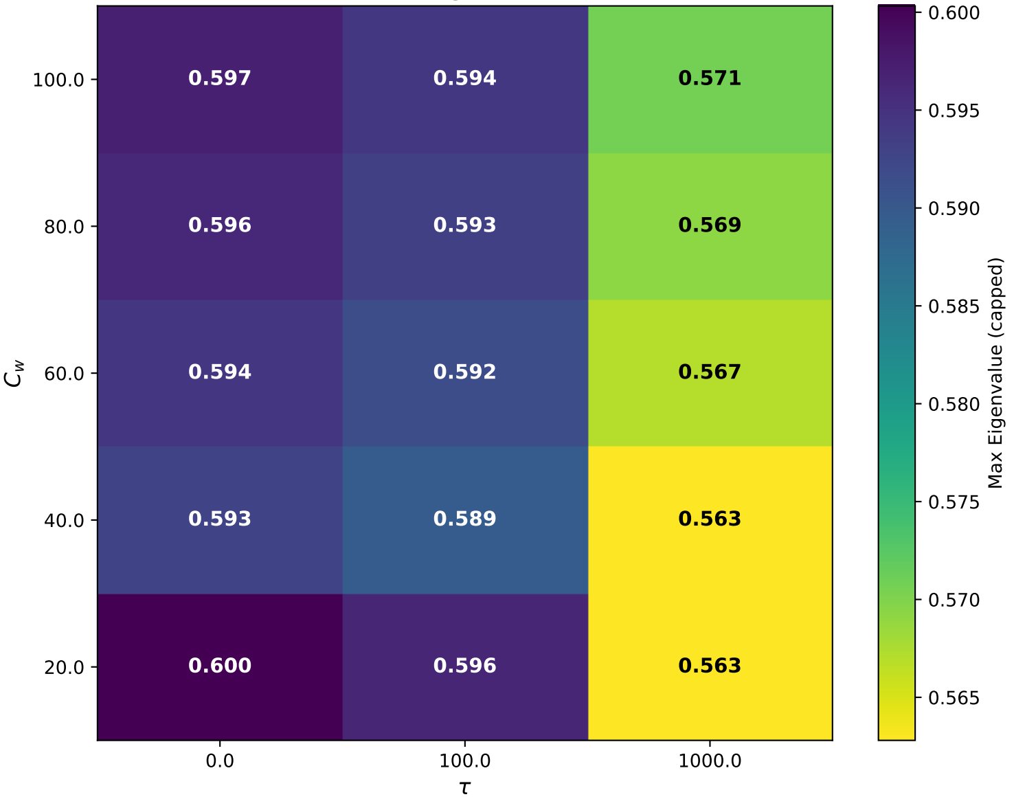
Max Eigenvalue
