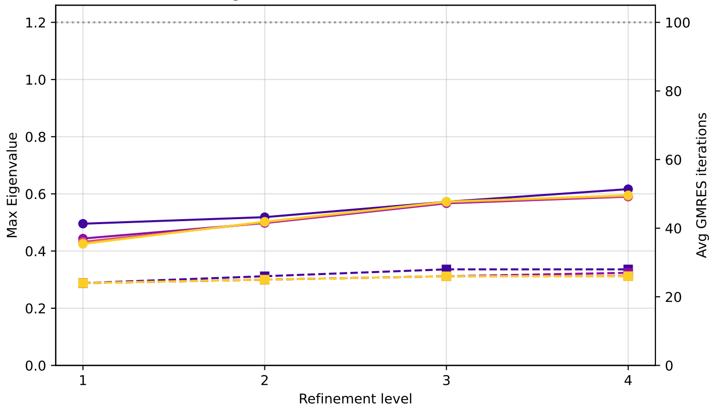
Eigenvalues and GMRES iterations
