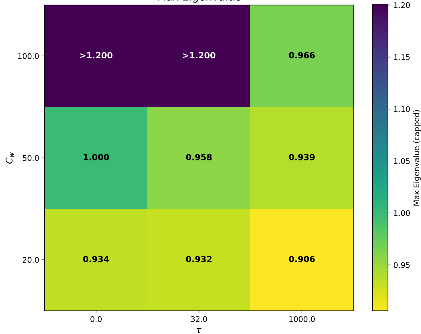
Max Eigenvalue
