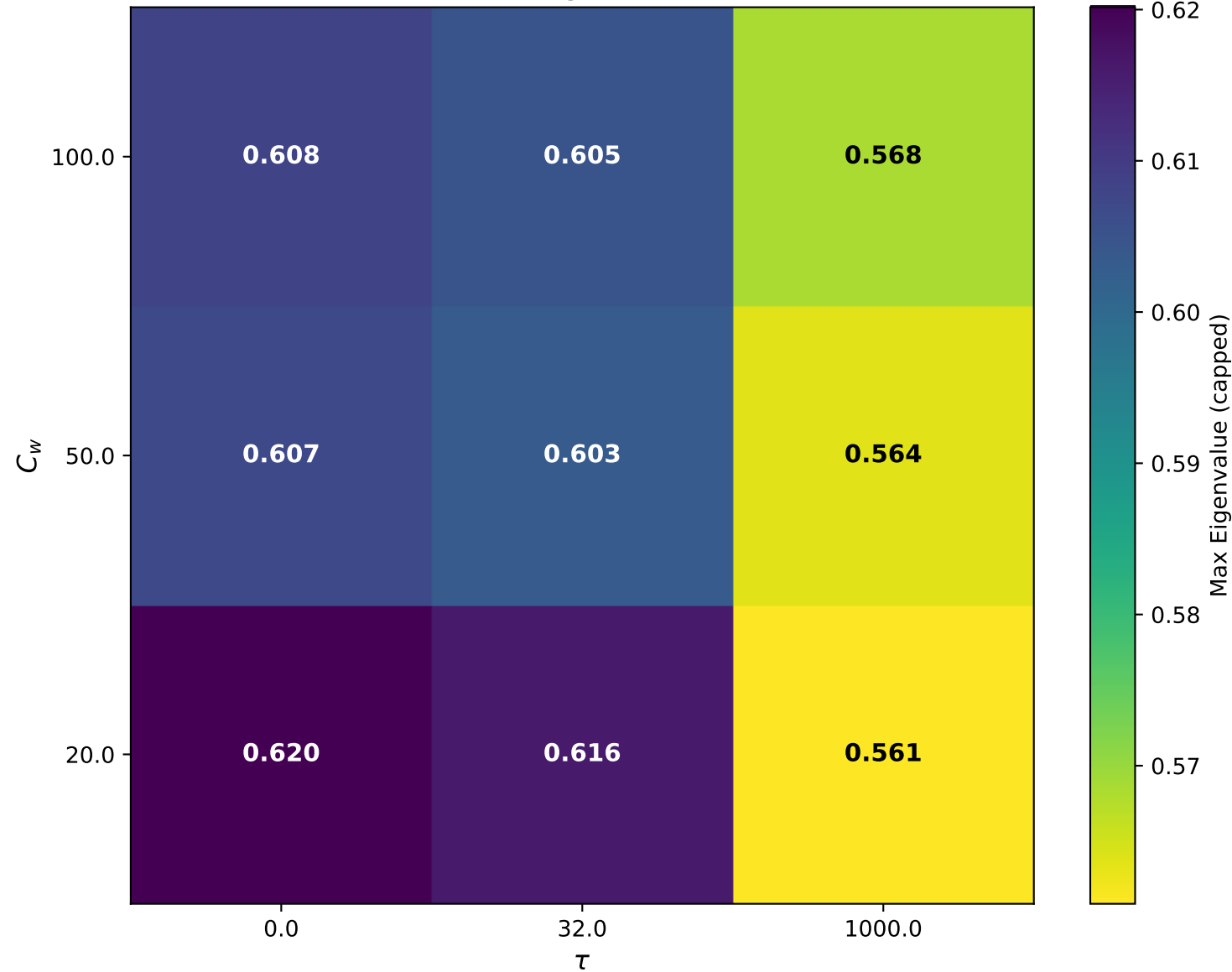
Max Eigenvalue
