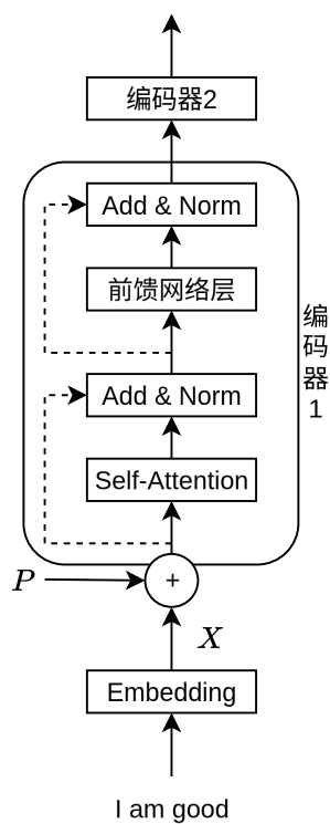
图 7.1: Transformer 编码器结构
