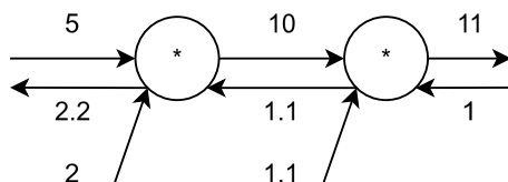
图 2.2: 反向传播示例
