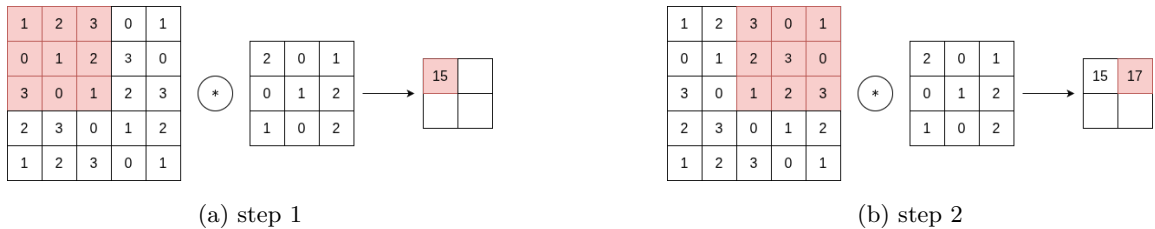
图 3.6: 步幅示例
