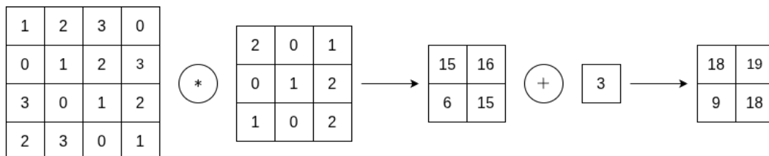
图 3.4: 偏置示例
