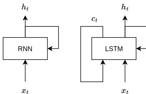
图 5.3: RNN 与 LSTM
