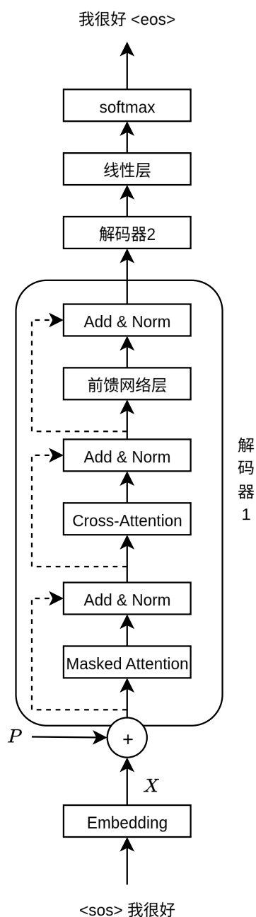
图 7.2: Transformer 解码器结构
