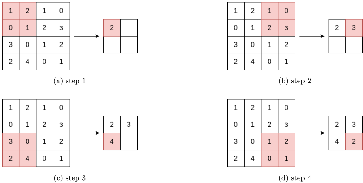
图 3.7: 池化层流程说明
