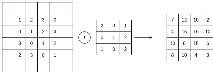
图 3.5: 填充示例
