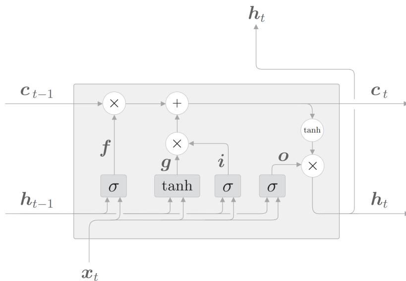
图 6.4: LSTM 的计算过程
