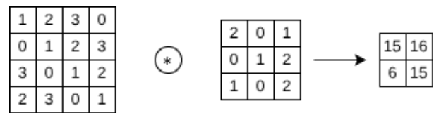
图 3.3: 卷积运算示例
