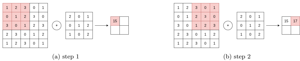
图 3.7: 步幅示例
