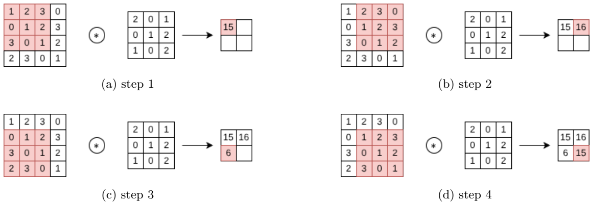
图 3.4: 卷积运算流程说明
