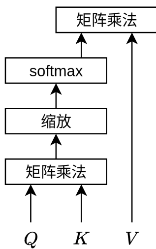
图 7.2: 自注意力计算流程
