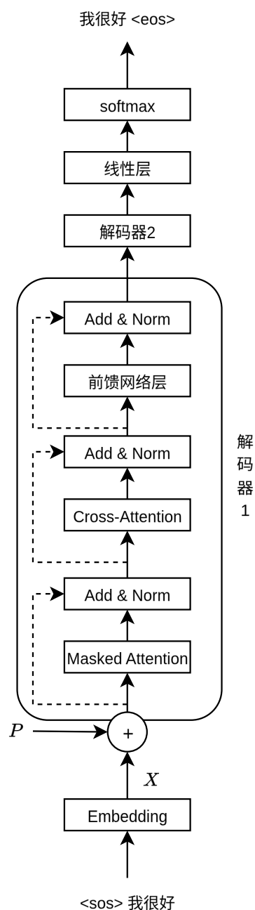
图 8.2: Transformer 解码器结构
