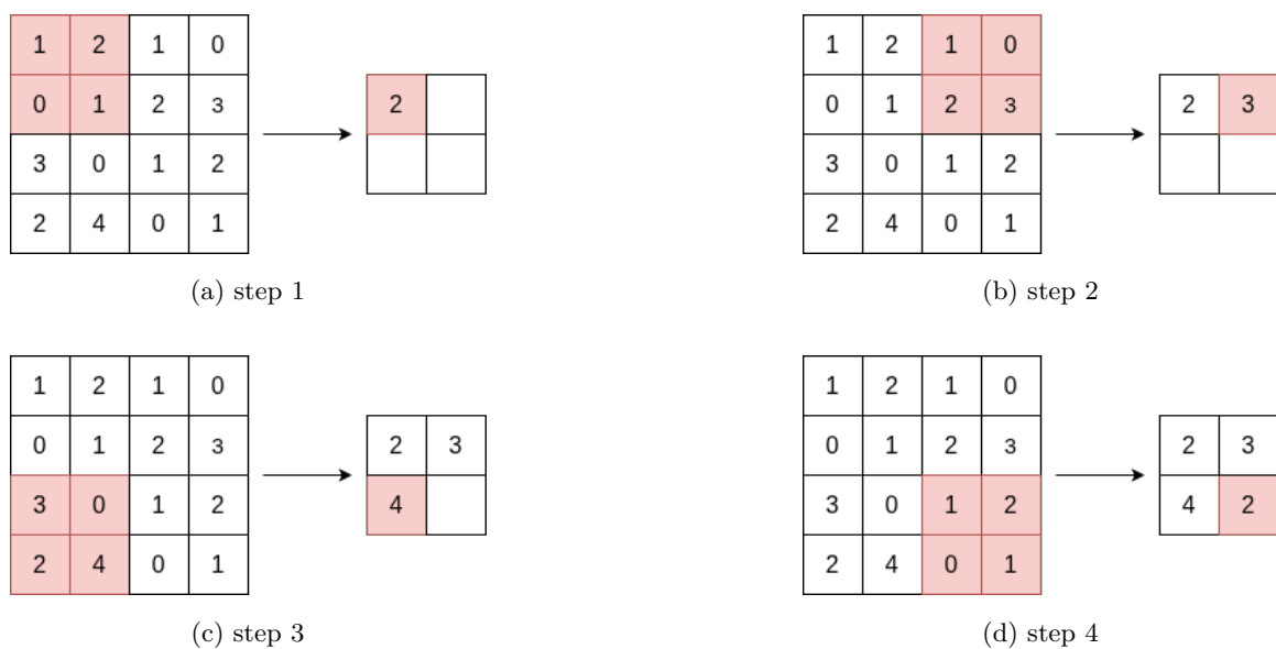
图 3.8: 池化层流程说明
