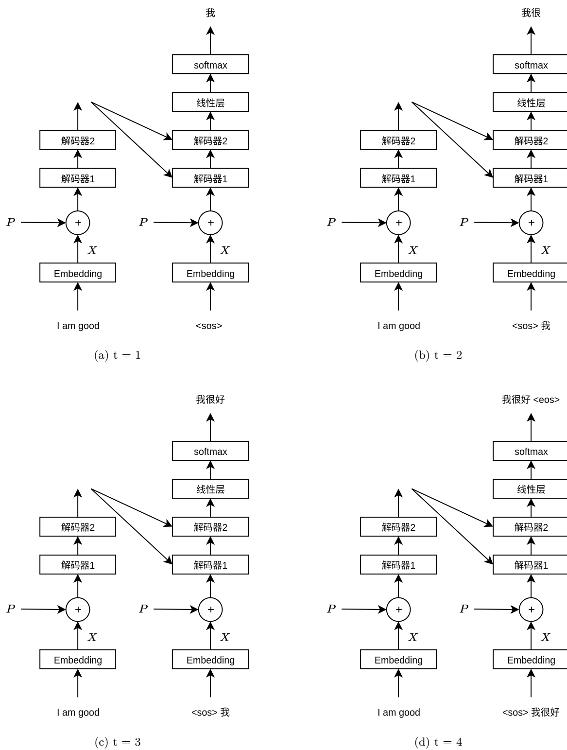
图 8.3: 解码器流程说明
