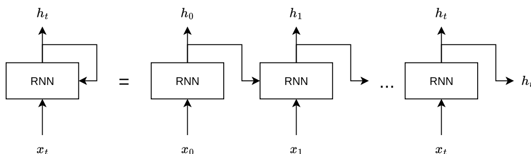
图 6.2: RNN 的展开
