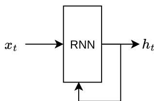
图 6.1: RNN 层示例
