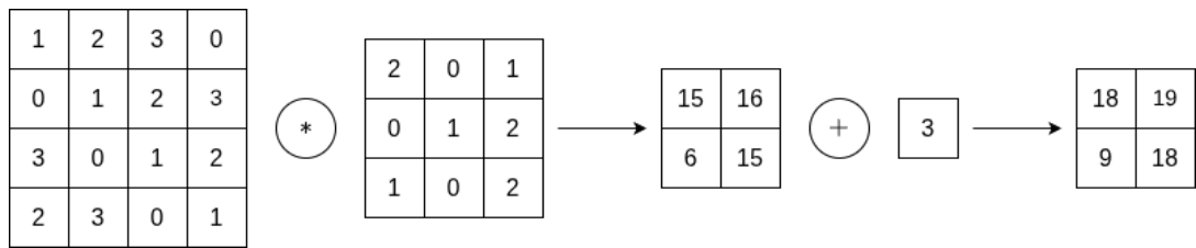
图 3.5: 偏置示例
