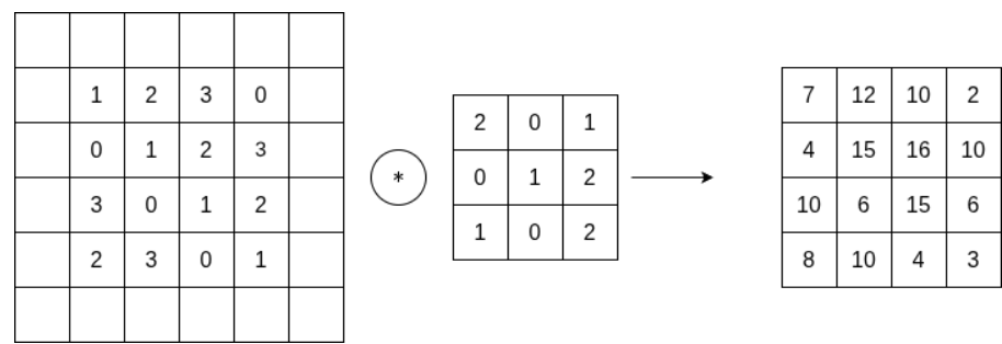
图 3.6: 填充示例
