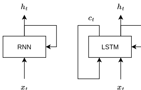
图 6.3: RNN 与 LSTM
