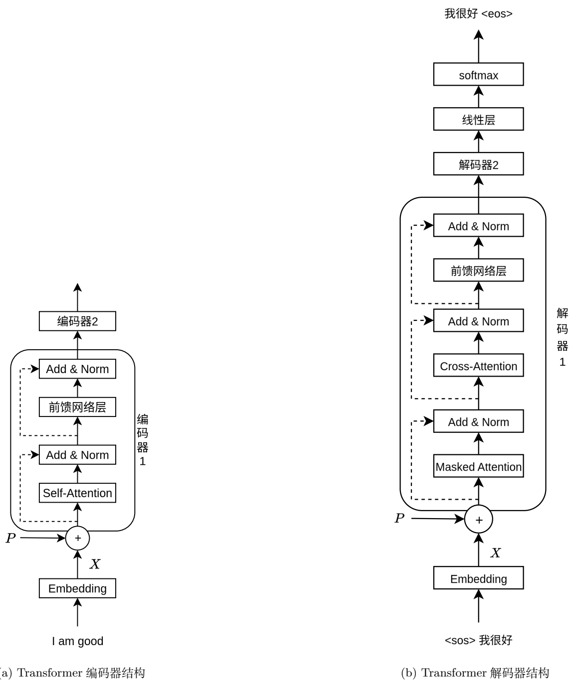
图 6.3: Transformer 结构
