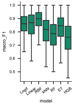
Macro-F1
