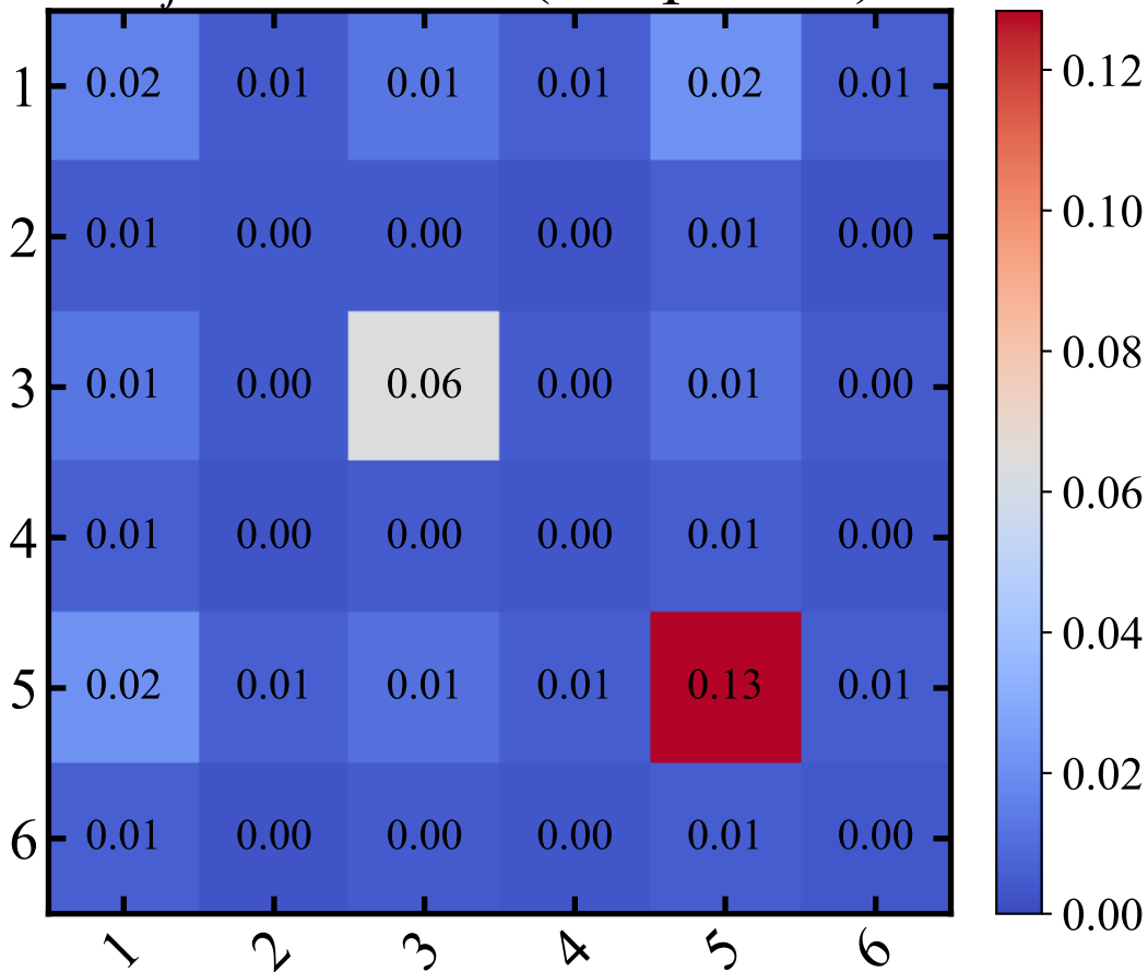
a_{ij} — NbTaTi (sample 1/1)
