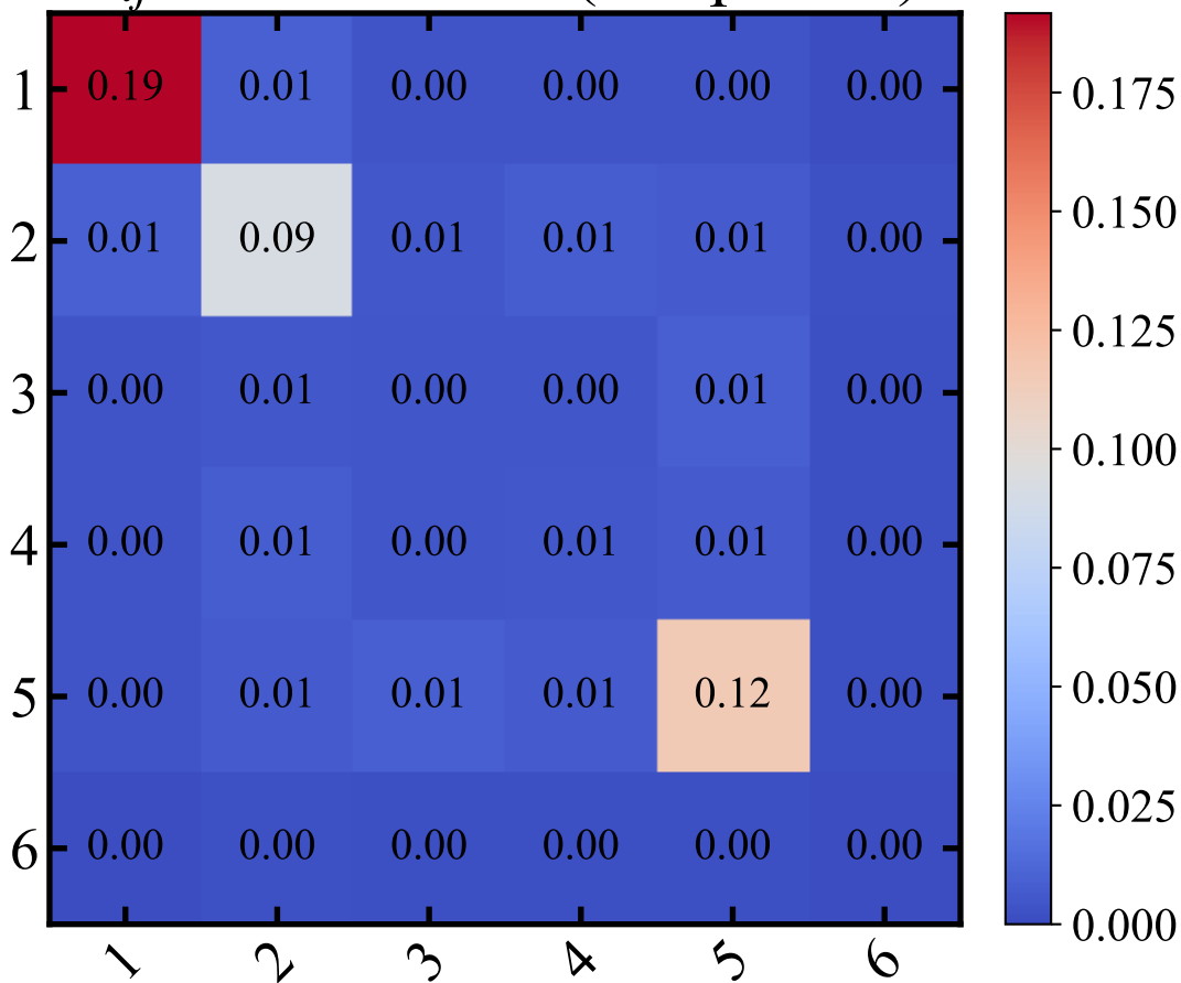
a_{ij} — HfNbTaTi (sample 6/9)
