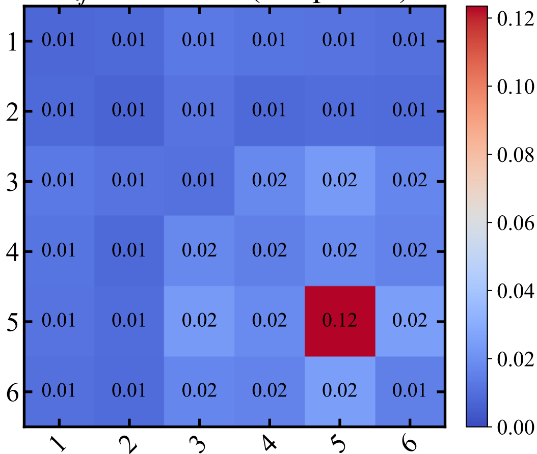
a_{ij} — HfNbTi (sample 5/7)
