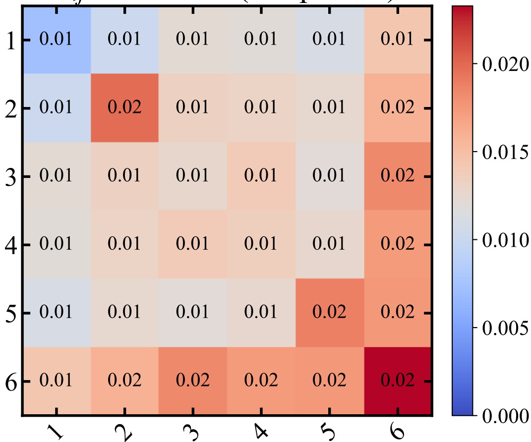
a_{ij} — NbTiZr (sample 5/8)
