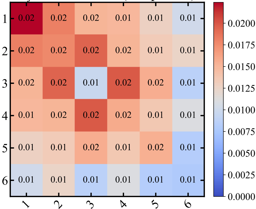
a_{ij} — HfNbTaTi (sample 9/9)
