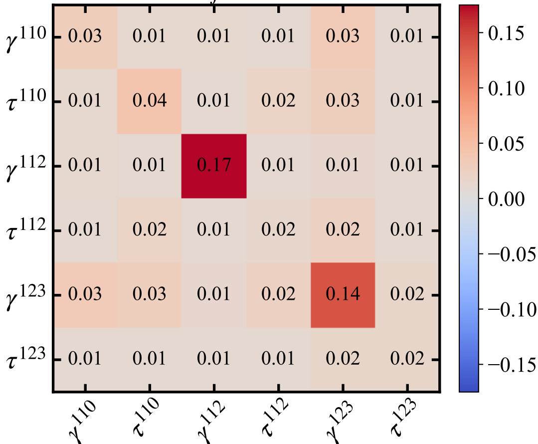
Mean a_{ij} over dataset
