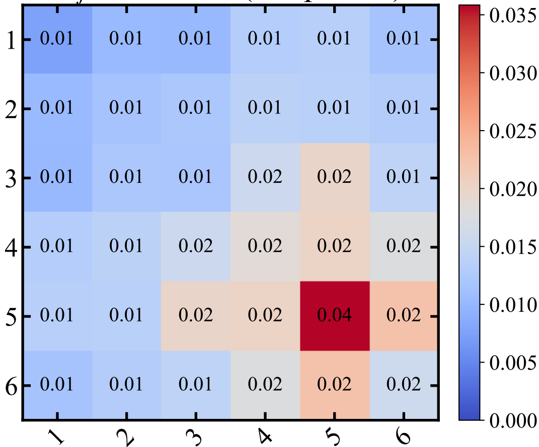
a_{ij} — NbTiZr (sample 6/8)
