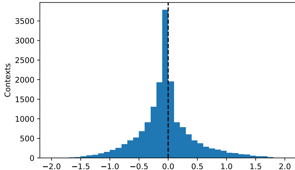
kendall: FLASH minus Baseline
