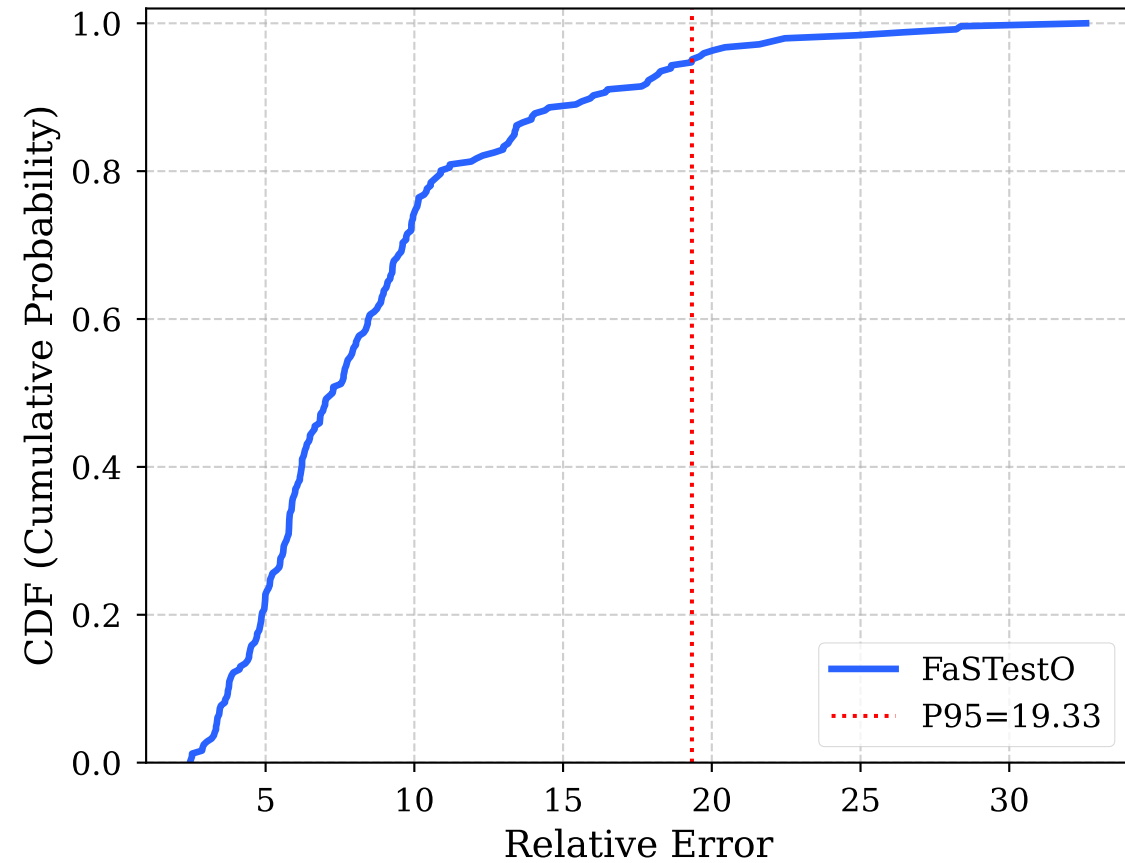
Error CDF
