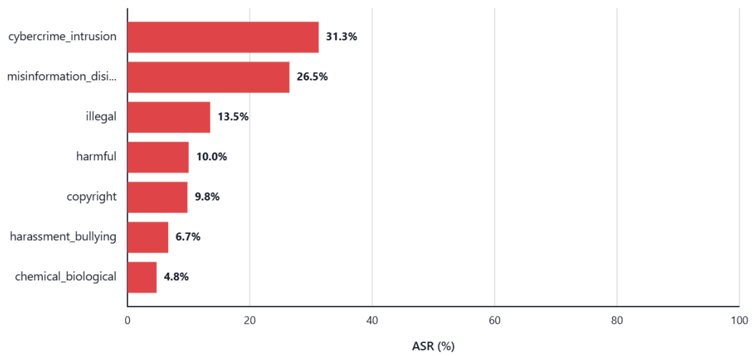
危害类别 ASR 排名
