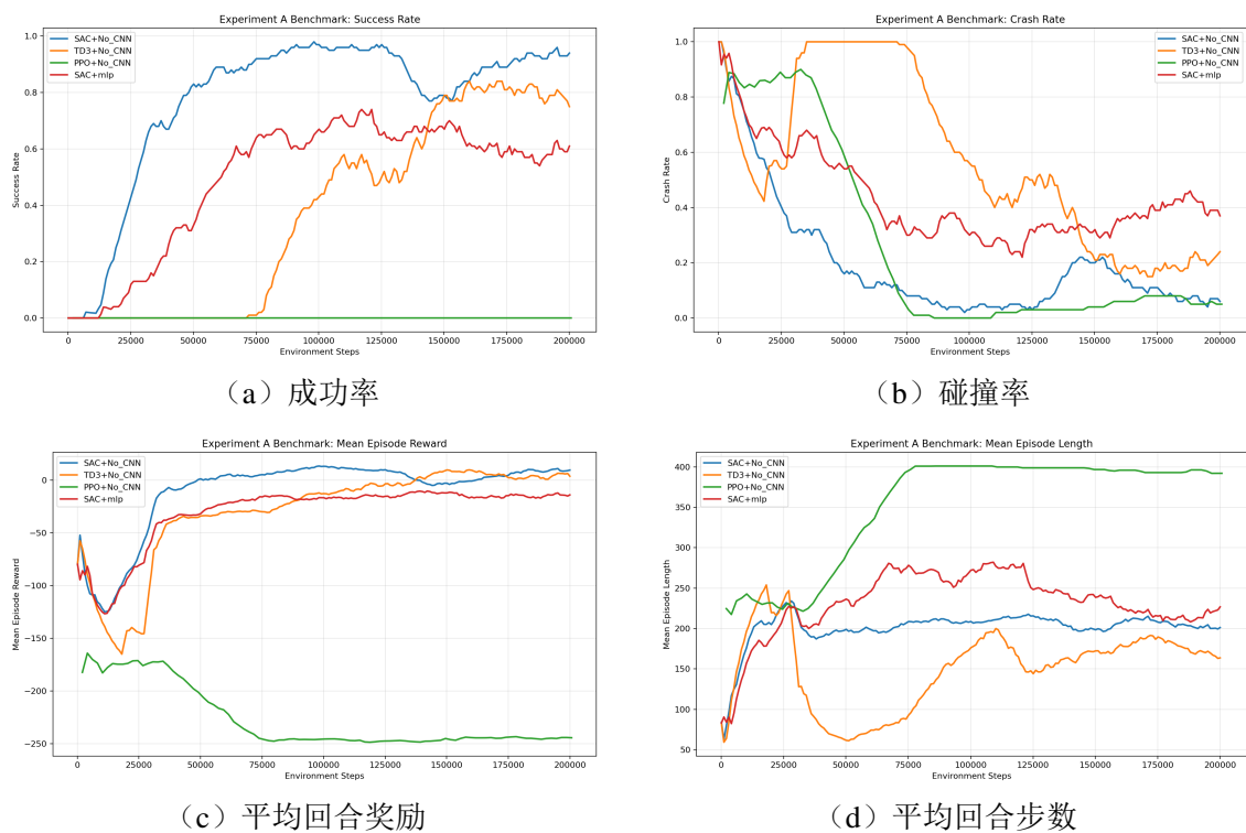
图 6: 四种配置训练 rollout 指标曲线
