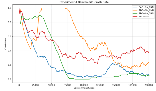
(b) 碰撞率
