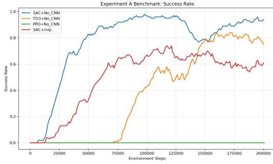
(a) 成功率
