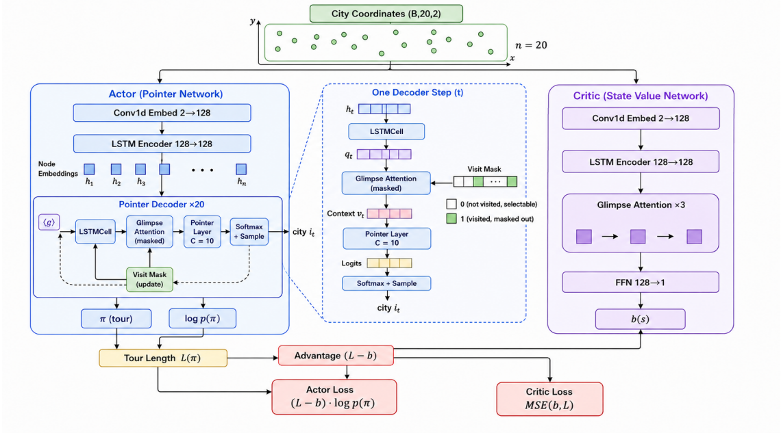
图 4: 指针网络 TSP 训练架构 (Actor-Critic REINFORCE)
