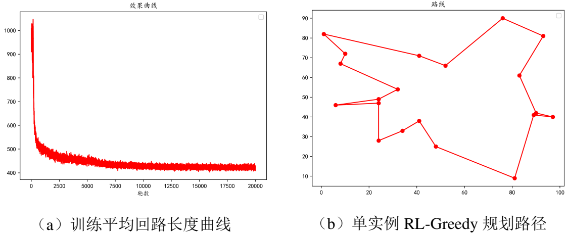
图 3: 指针网络 TSP 训练过程与单实例路径可视化 ( n = 20 )
