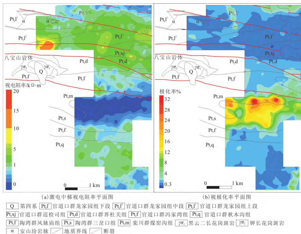
图 6 激电中梯视电阻率平面图和视极化率平面图
