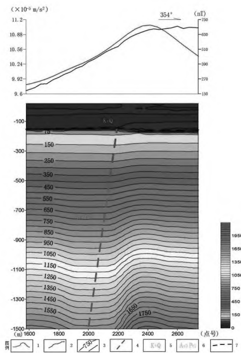
图2 园宅集DC-y1异常区综合物探剖面图
