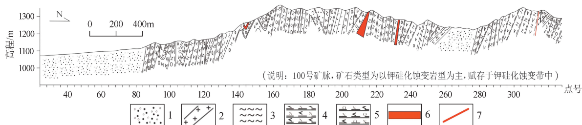
图 5 大坝沟东侧 100 号矿脉露头实测地质剖面图
