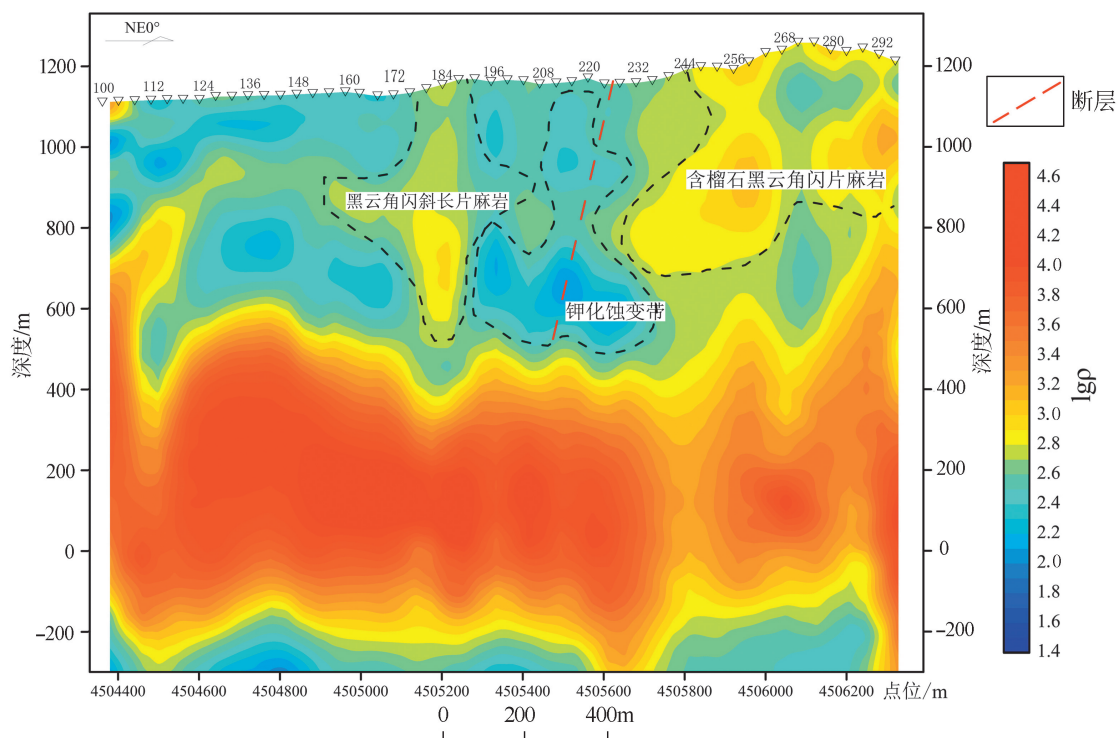
图 6 研究区 900 线 CSAMT 二维反演电阻率等值线断面图及推断构造
