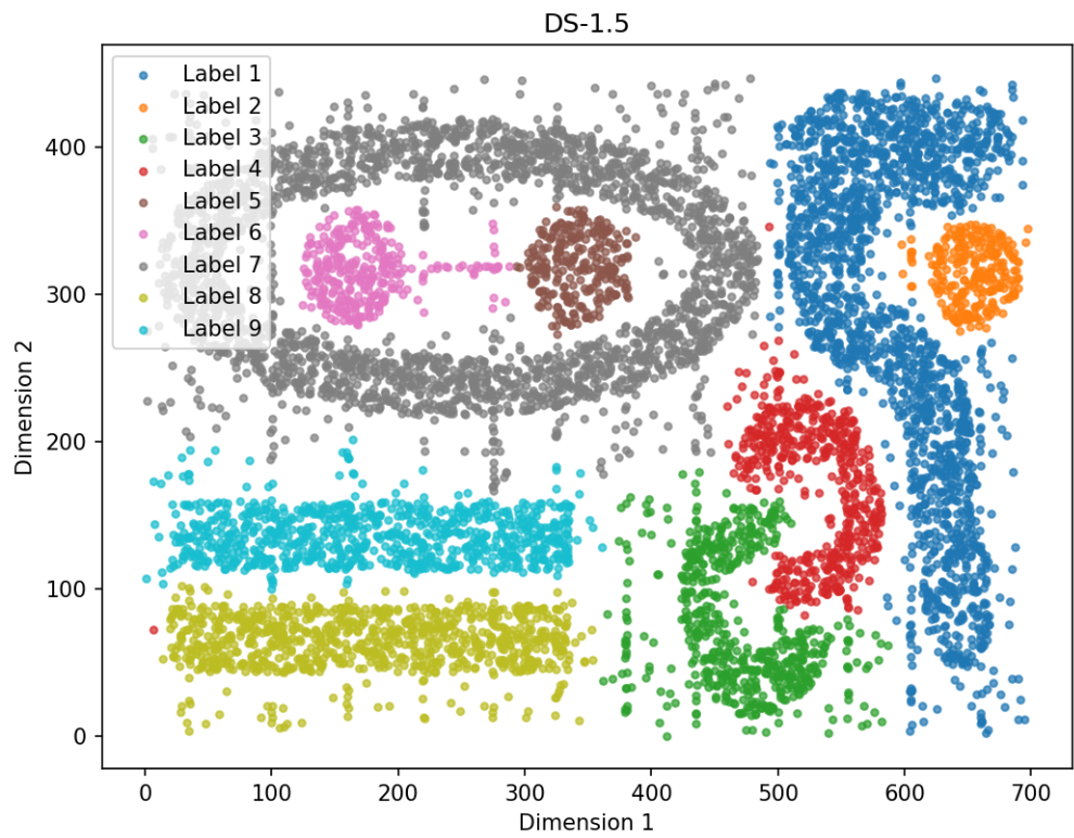
图4.8 DS-1.5上的聚类结果
