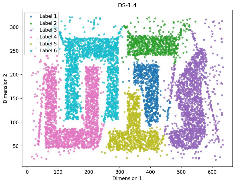
图4.7 DS-1.4上的聚类结果
