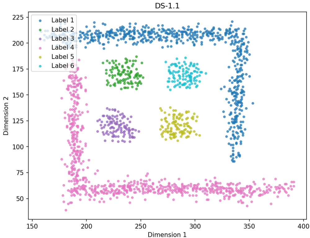
图4.4 DS-1.1上的聚类结果
