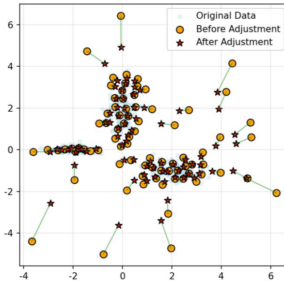
图3.2 代表点位置调整前后示意图
