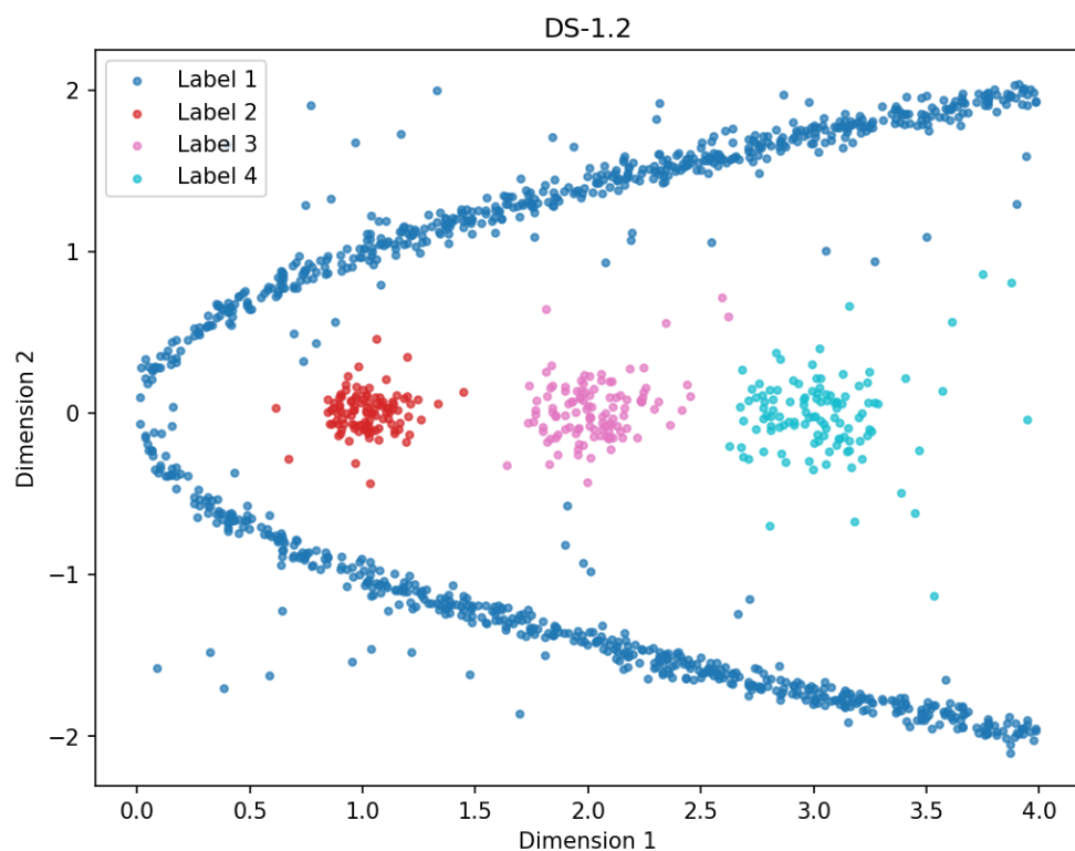
图4.5 DS-1.2上的聚类结果
