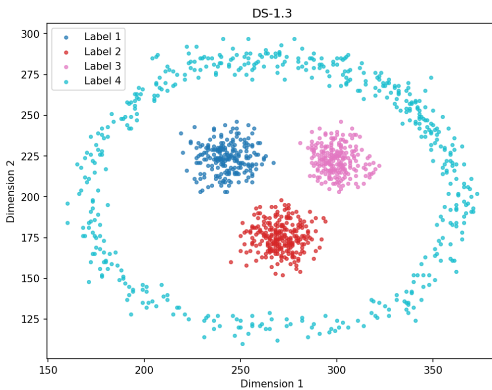
图4.6 DS-1.3上的聚类结果
