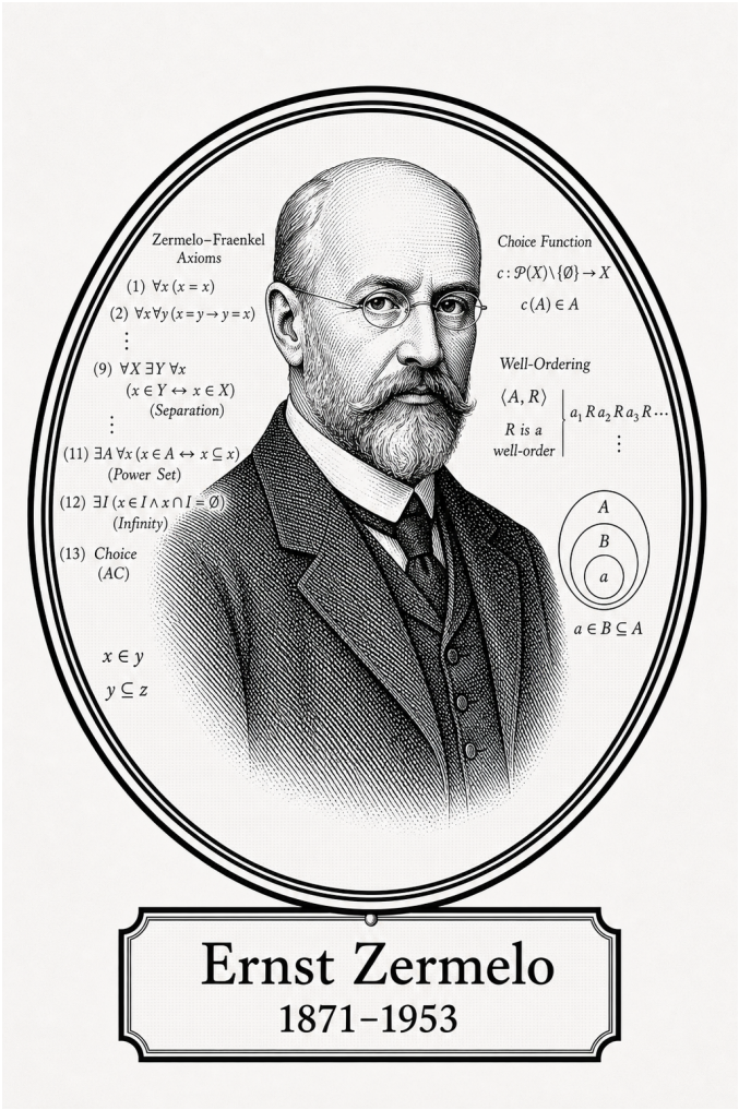
Ernst Zermelo
