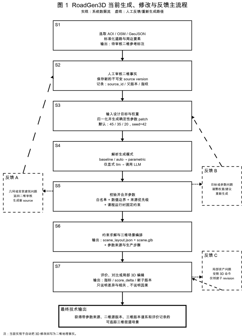
图 1 将“修改的触发—依据—执行位置—输出结果”串成一条可审计链。三条虚线回路是不同含义的反馈：几何问题回到 2D；目标问题回到参数输入；局部资产问题只创建 3D 子版本。
