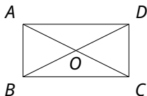
图 3.2-2 一个矩形
