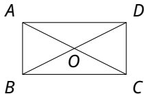
图 3.2-2 一个矩形
