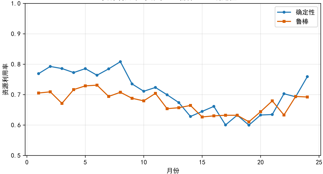
资源利用率跨期对比（鲁棒 vs. 确定性）
